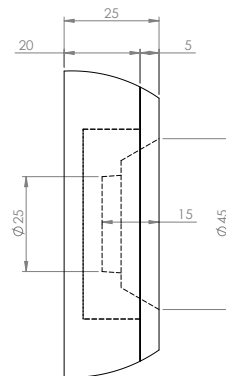
DÉTAIL A ECHELLE 1 : 1 DETAIL A SCALE 1 : 1
